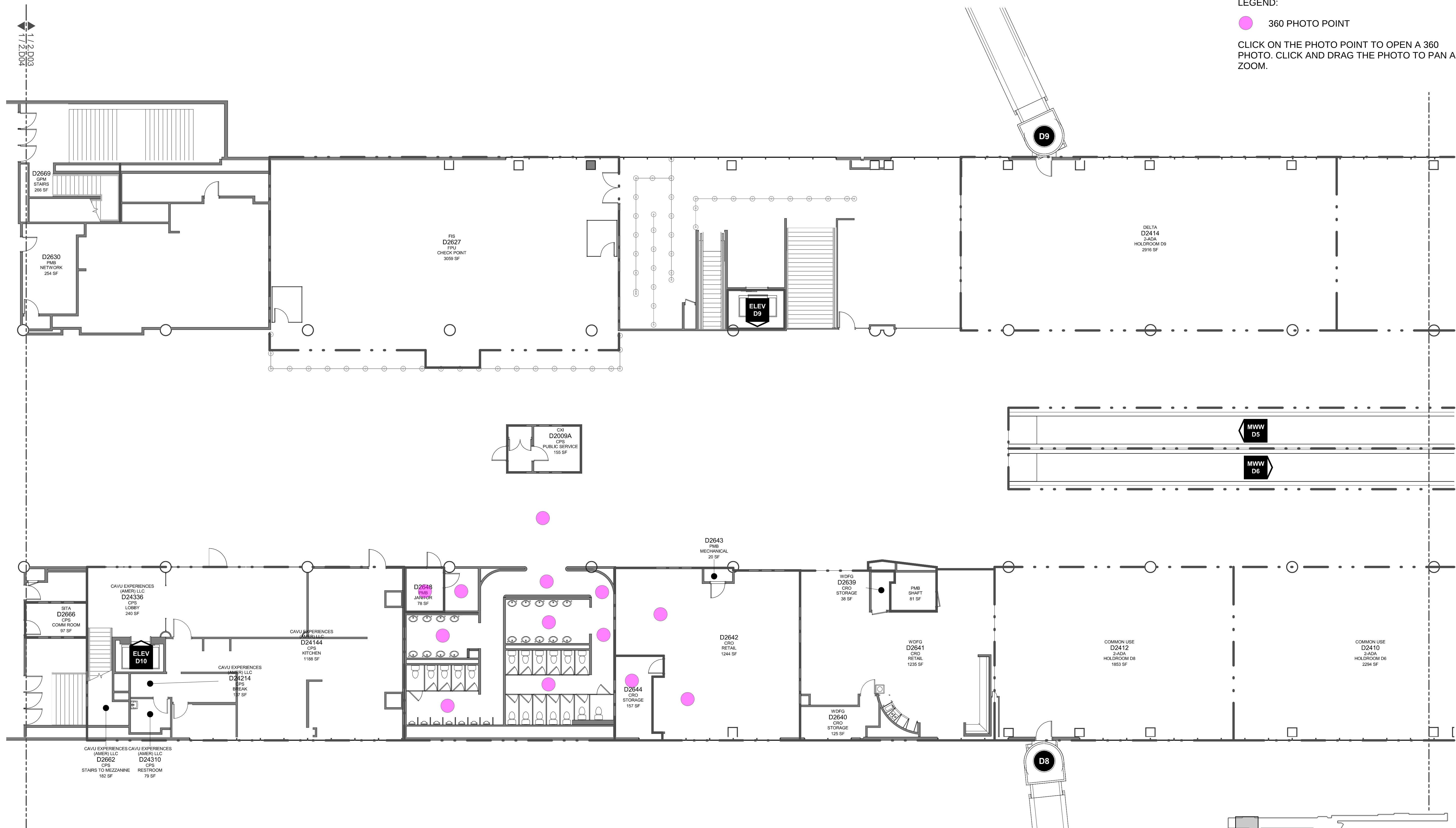
1 CONCURSE D - SECTOR 3 - D2646, D2647 - ENPLANING SCALE: 1" = 10'-0"
