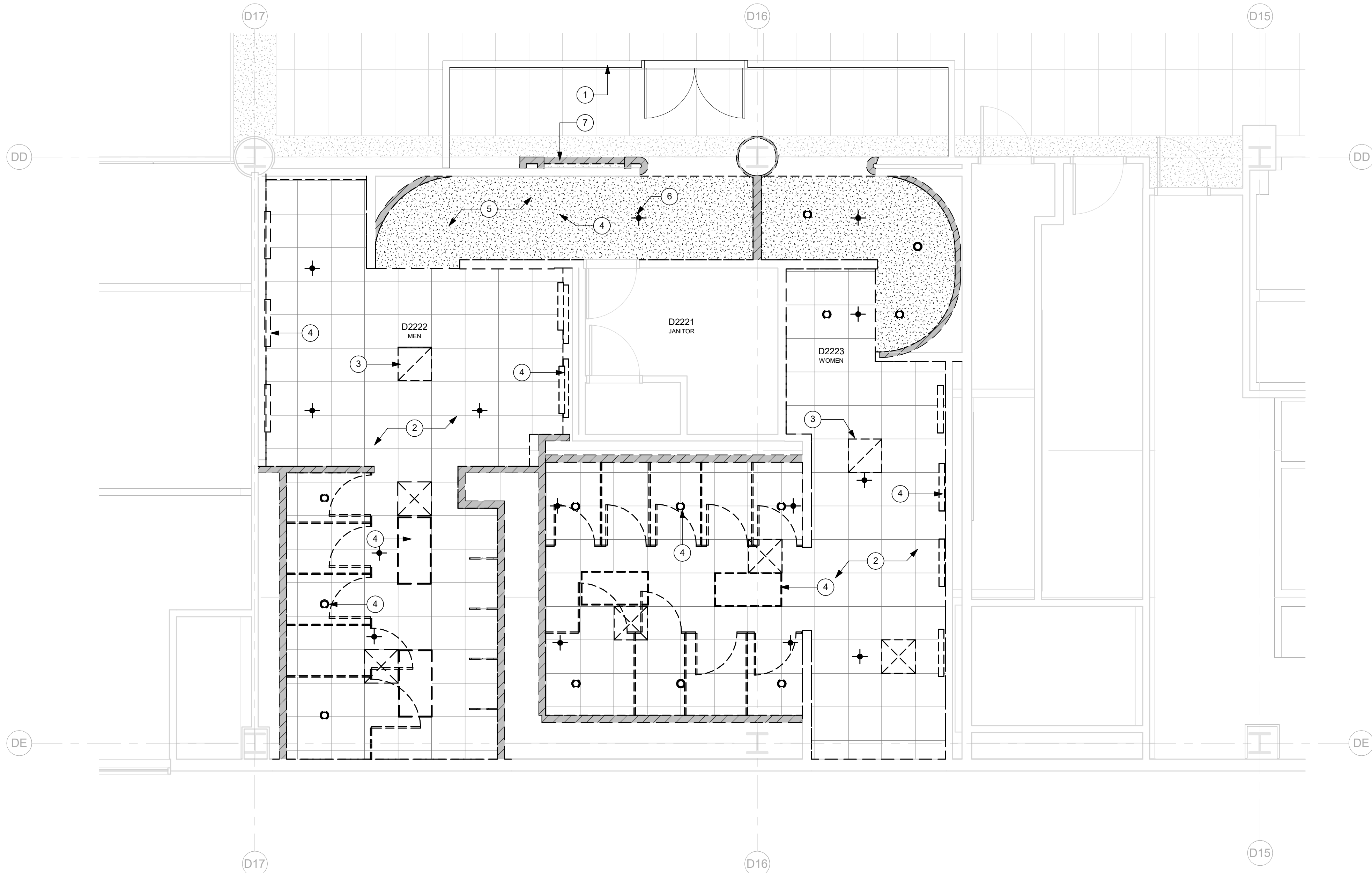
1 CONCURSE D - SECTOR 2 - D2221, D2222, D2223 - ENPLANING - DEMO RCP SCALE: 1/4" = 1'-0"
