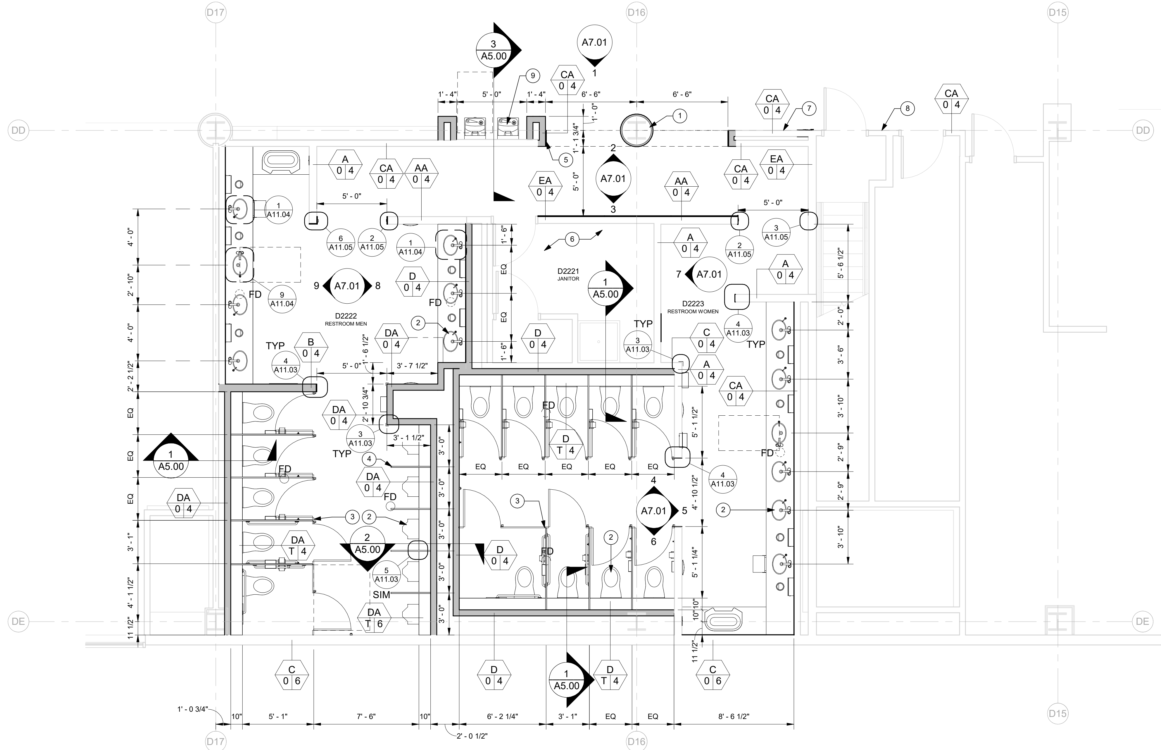
1 CONCURSE D - SECTOR 2 - D2221, D2222, D2223 - ENPLANING - FLOOR PLAN SCALE: 1/4" = 1'-0"
