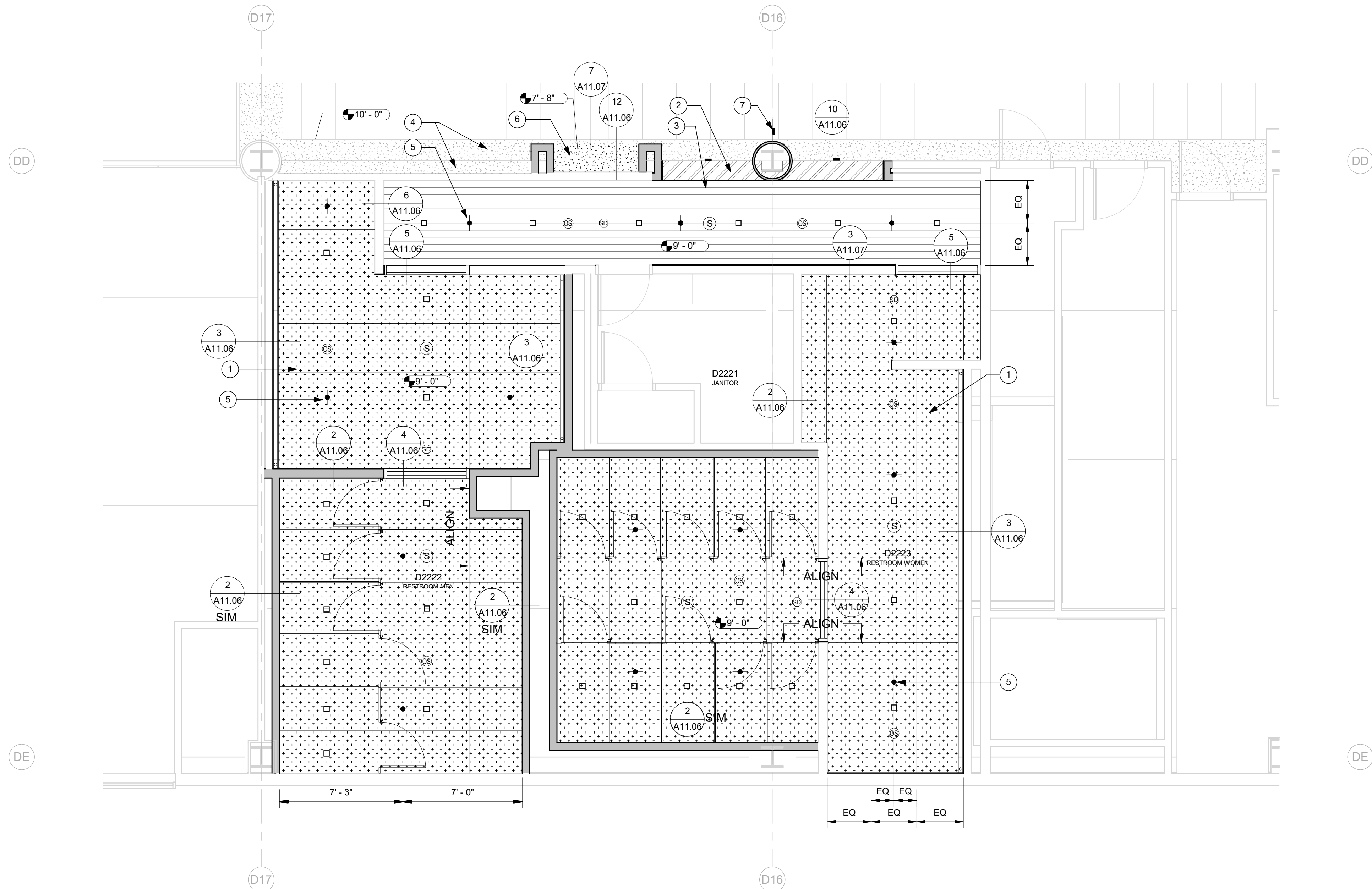
1 CONCURSE D - SECTOR 2 - D2221, D2222, D2223 - ENPLANING - RCP SCALE: 1/4" = 1'-0"
