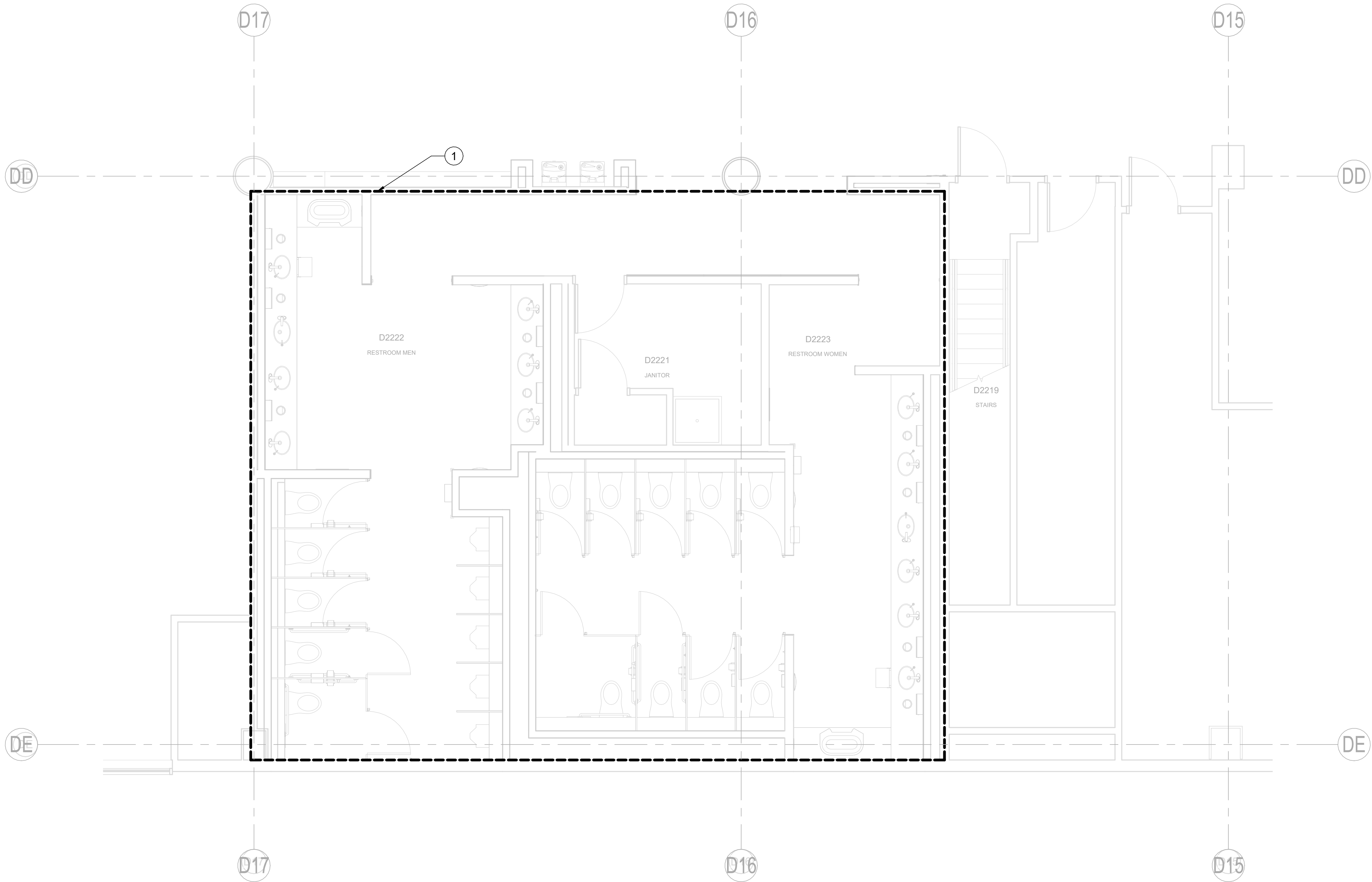
1 CONCOURSE D - SECTOR 2 - D2221, D2222, D2223 - ENPLANING - FLOOR PLAN - FIRE PROTECTION SCALE: 1/4" = 1'-0"
