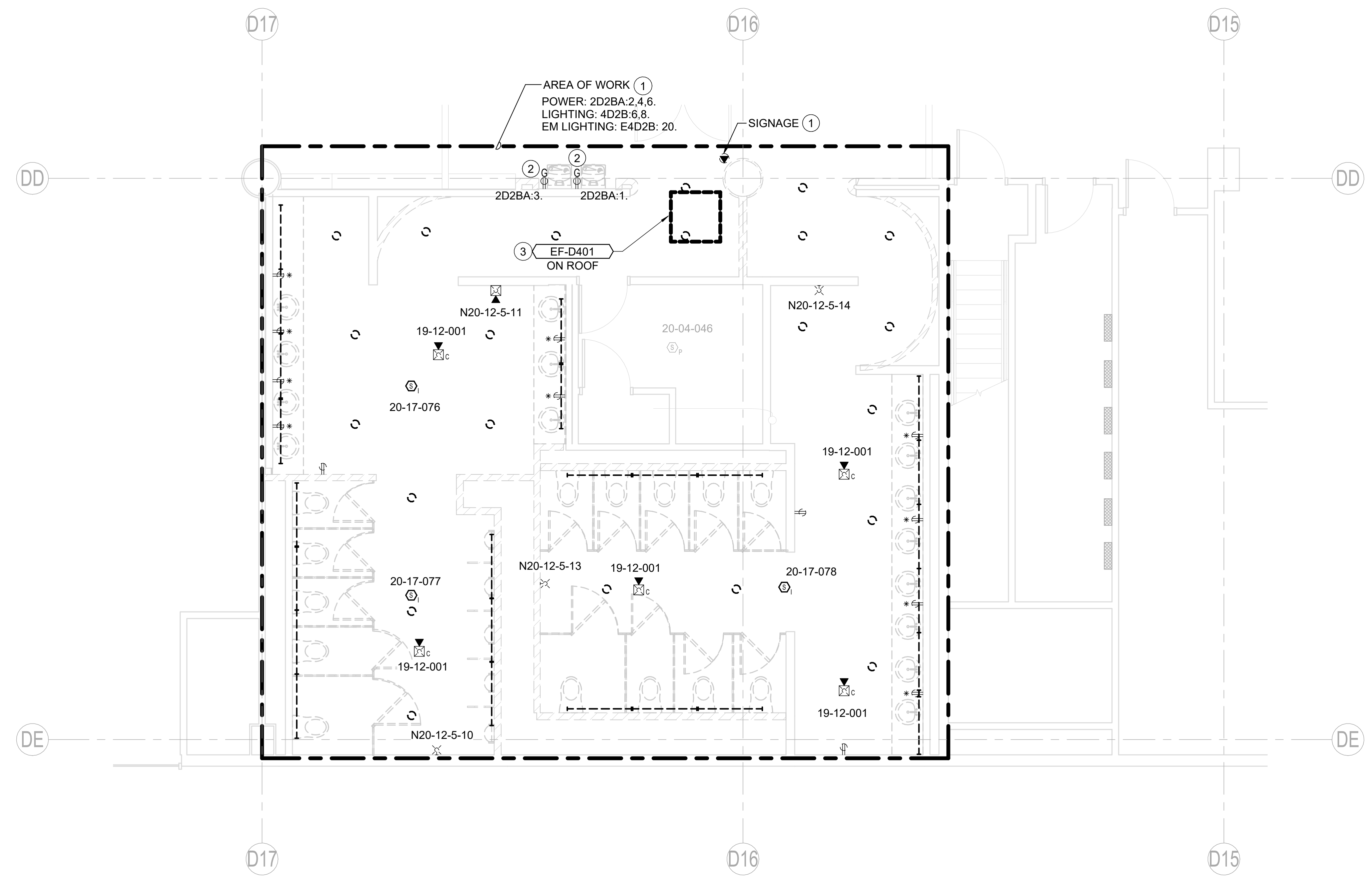
1 CONOURSE D - SECTOR 2 - D2221, D2222, D2223 - ENPLANING - DEMO PLAN - ELECTRICAL SCALE: 1/4" = 1'-0"
