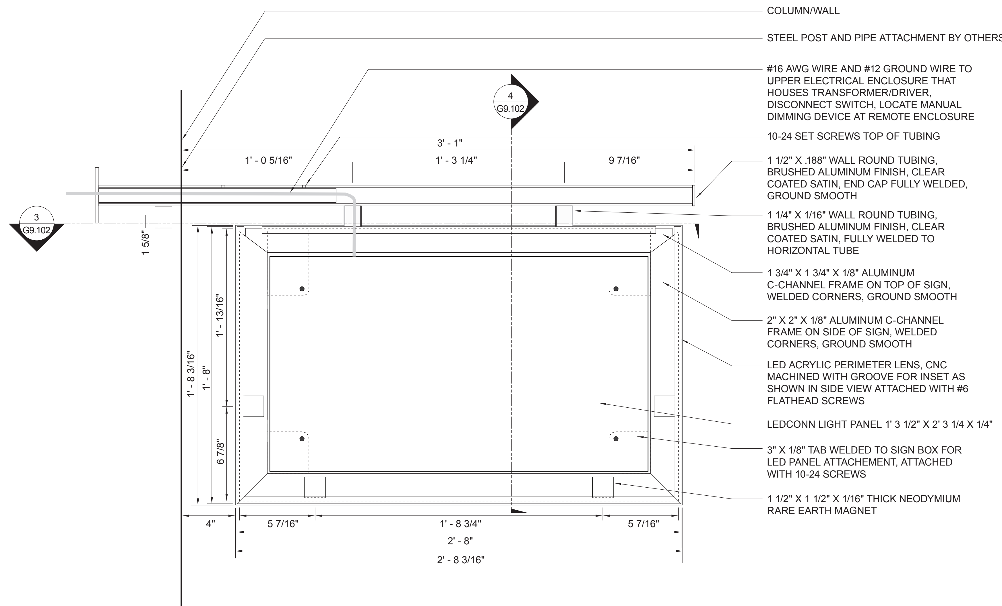
2 CBL - ELEVATION SCALE: 3\"/>
