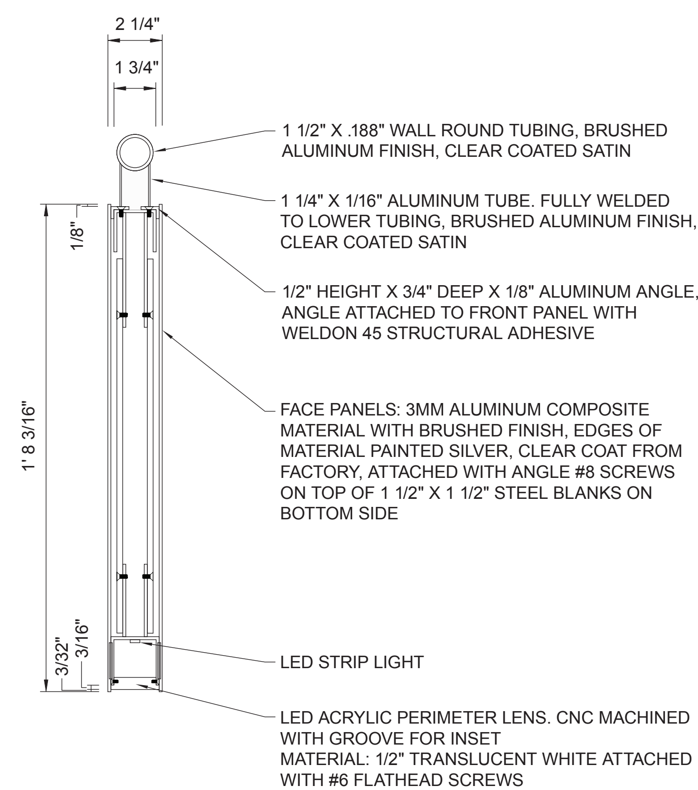
4 CBL - SECTION SCALE: 3\"/>
