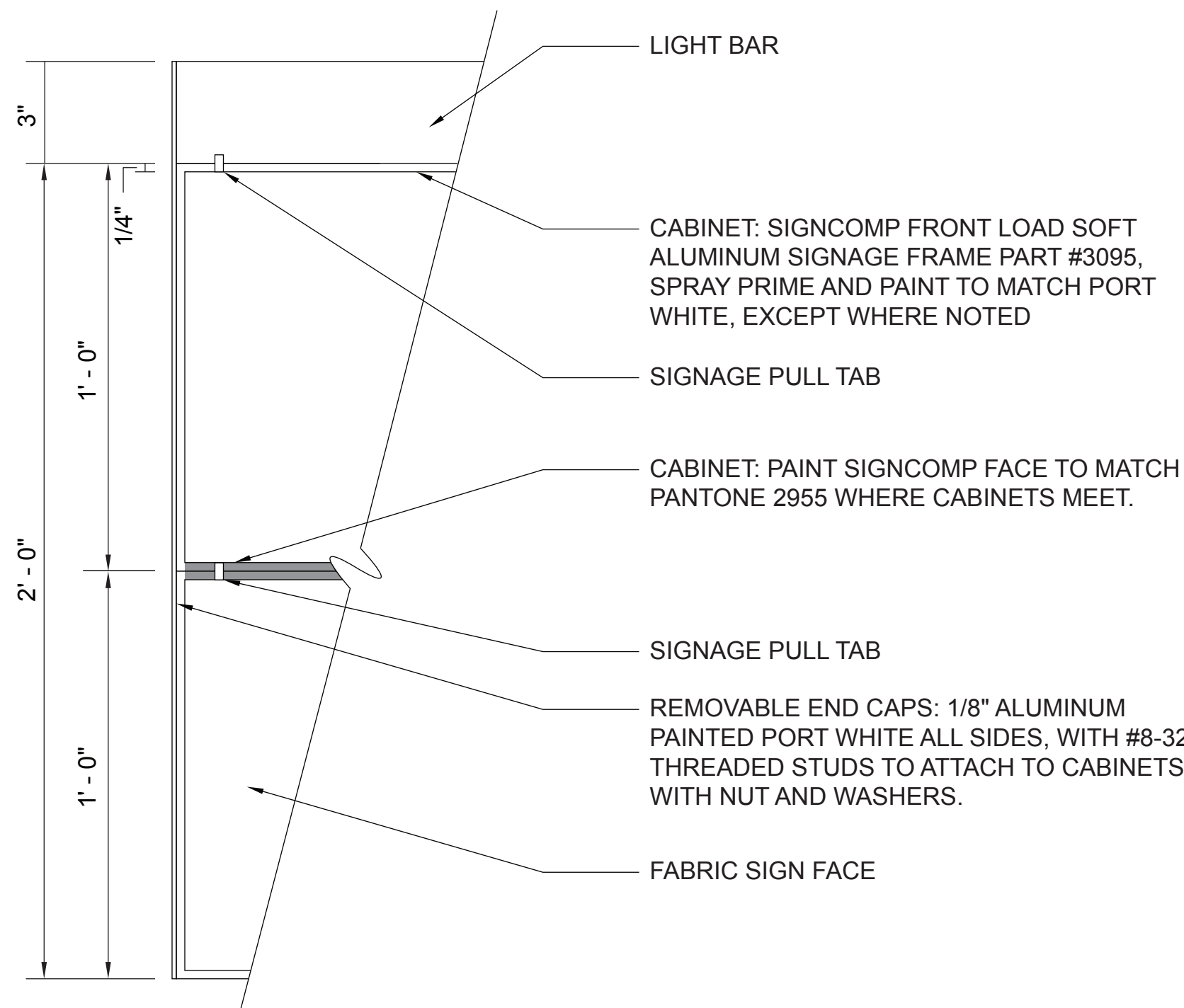
5 CM2 - DETAIL SCALE: 3" = 1' - 0"
