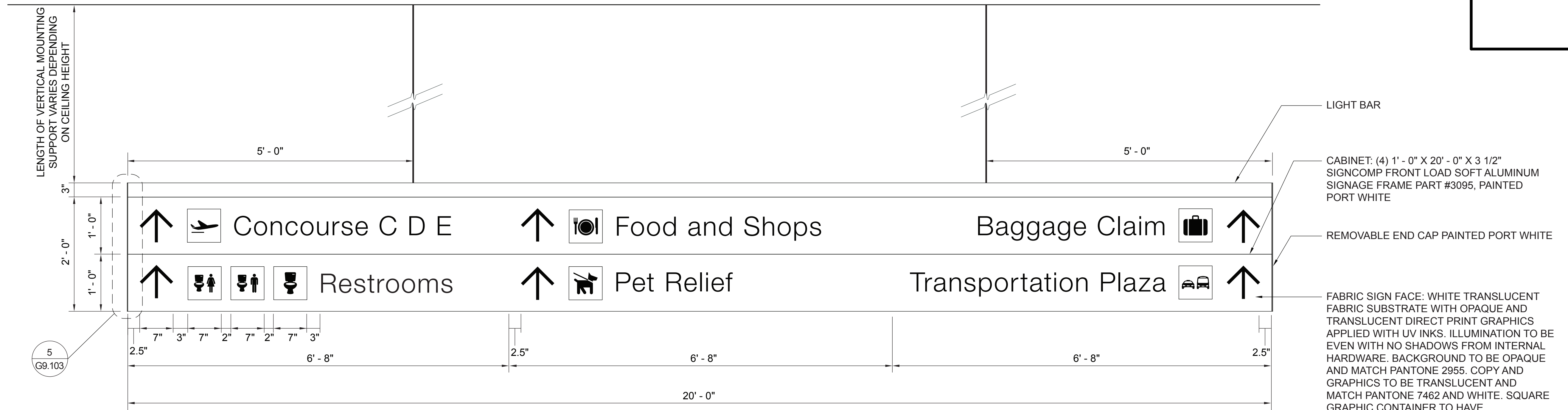
2 CM2 - ELEVATION SCALE: 1" = 1' - 0"
