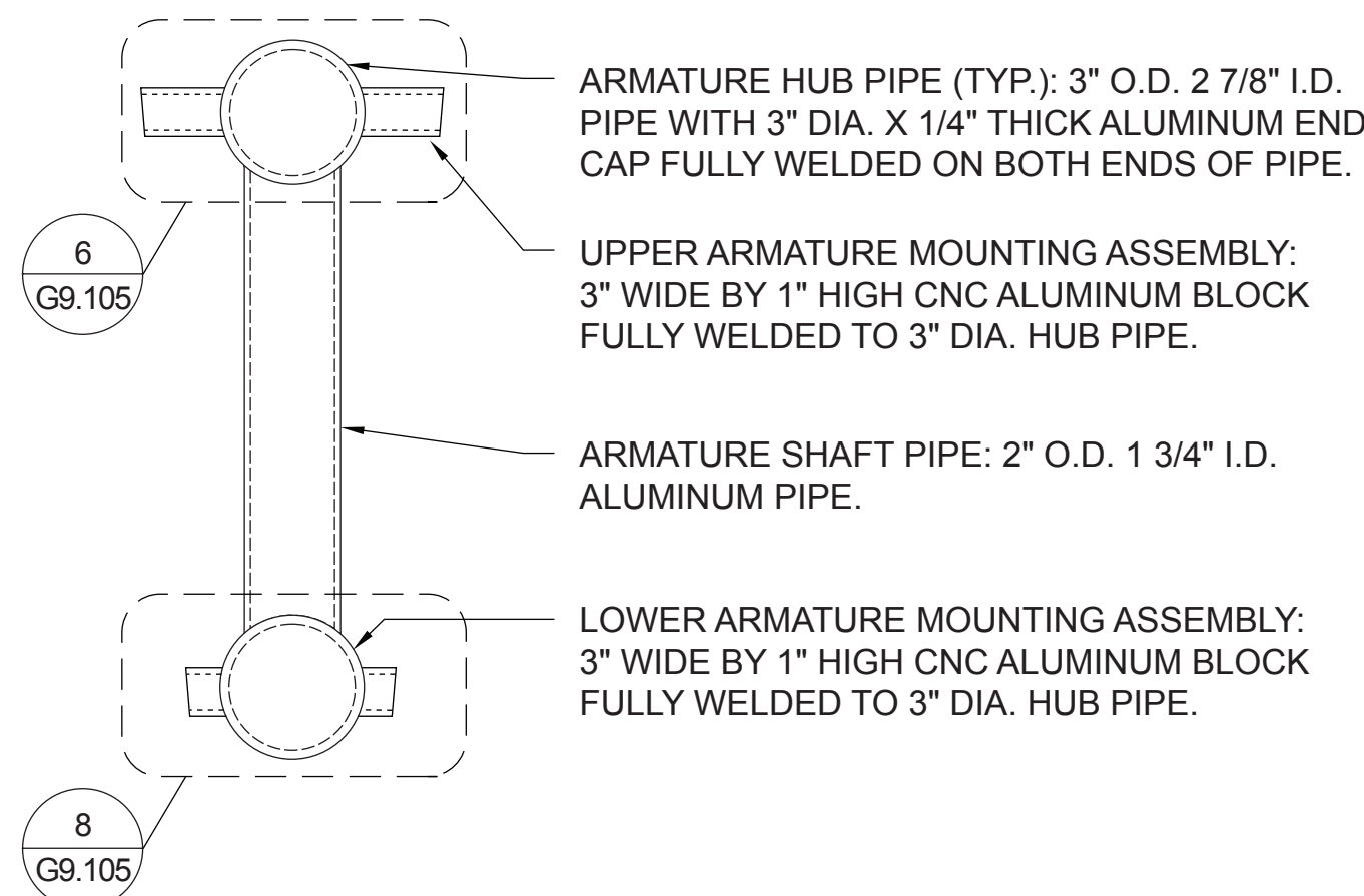
1 CM2 - ARMATURE SECTION SCALE: 3" = 1"
