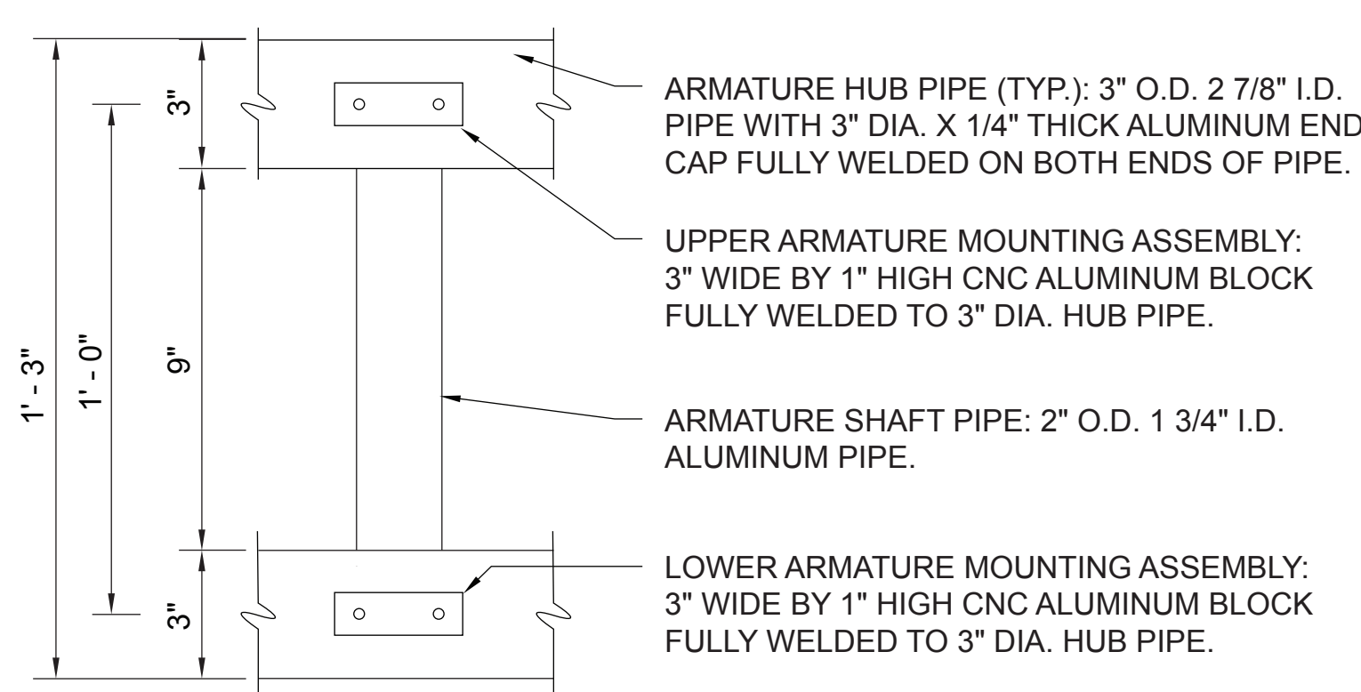
2 CM2 - ARMATURE ELEVATION SCALE: 3" = 1"
