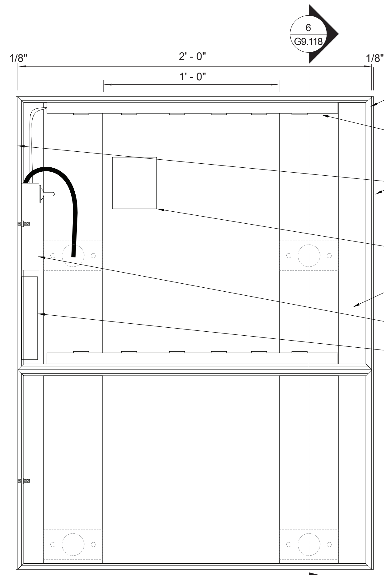
5 WM4 - ELEVATION SCALE: 3" = 1' - 0"
