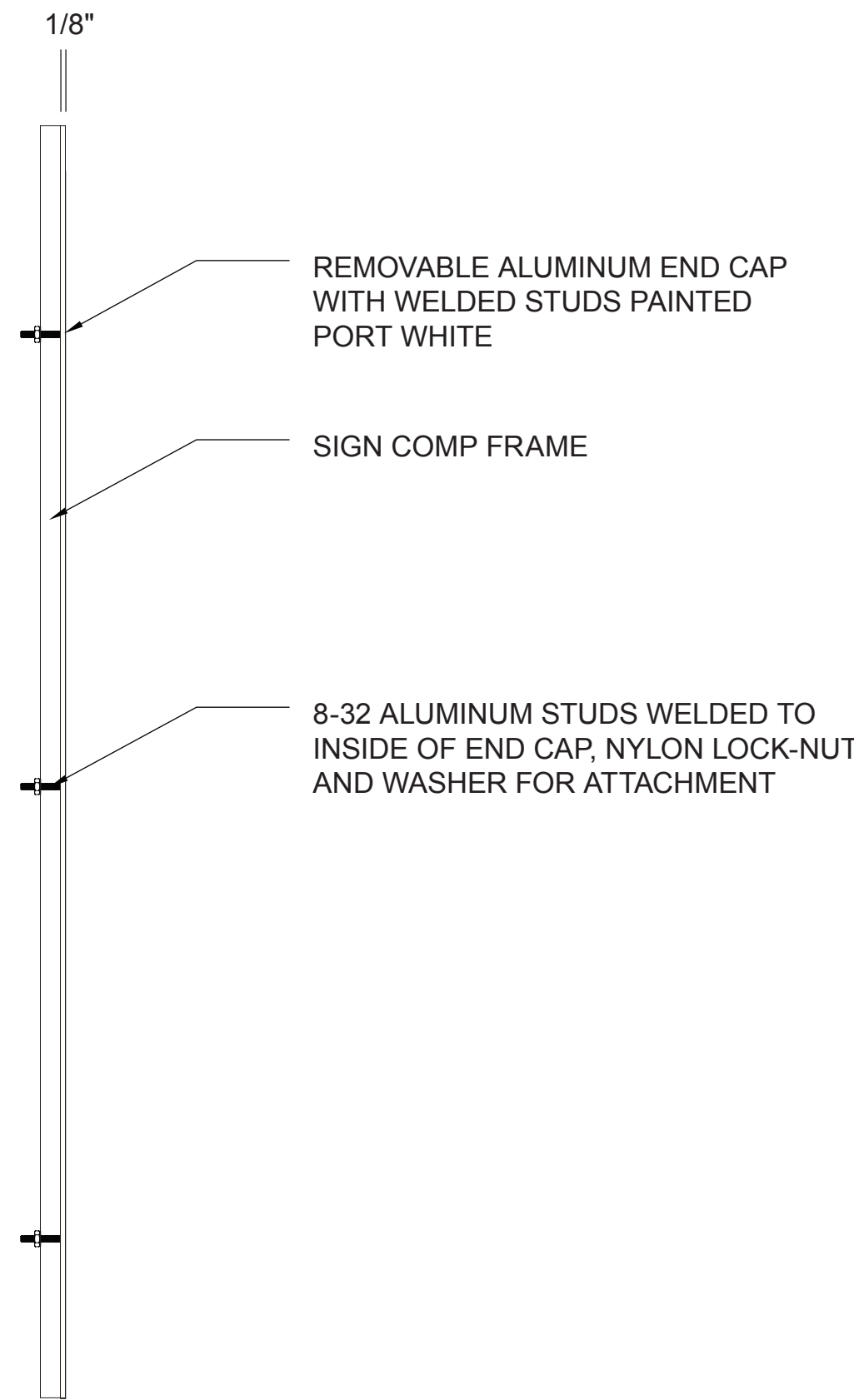
4 WM4 - END CAP SECTION SCALE: 3" = 1' - 0"
