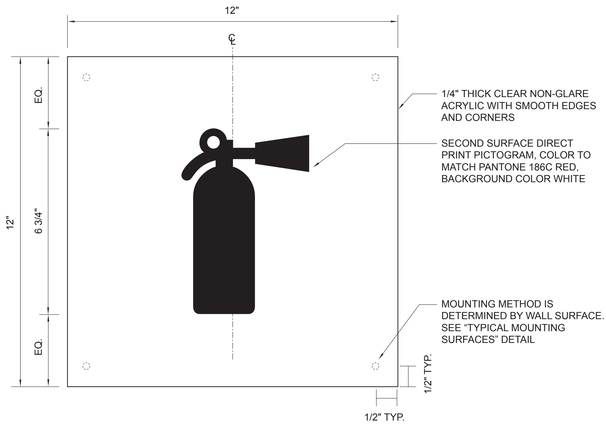
4 IFW - ELEVATION SCALE: HALF SIZE
