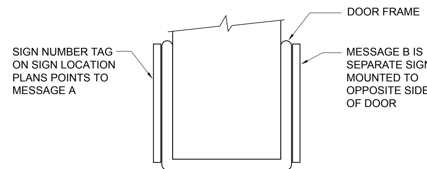
6 ID1 - SECTION SCALE: FULL SIZE
